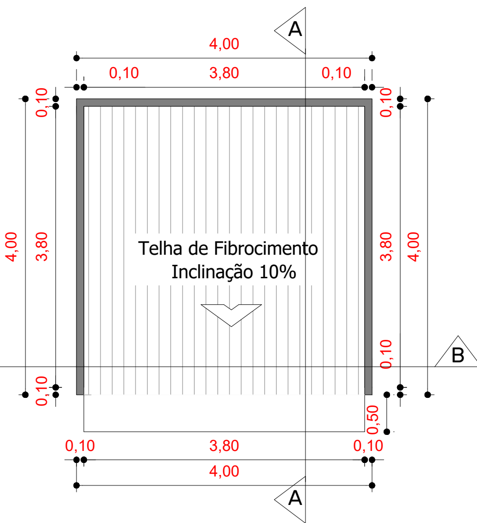
COBERTURA ESC. 1:50
