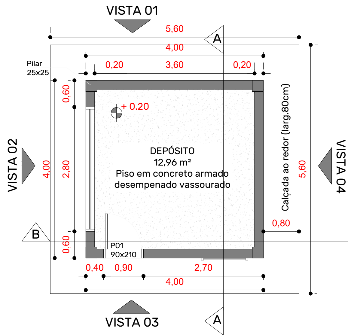
PLANTA - PAVI. TÉRREO (DEPÓSITO) ESC. 1:50
