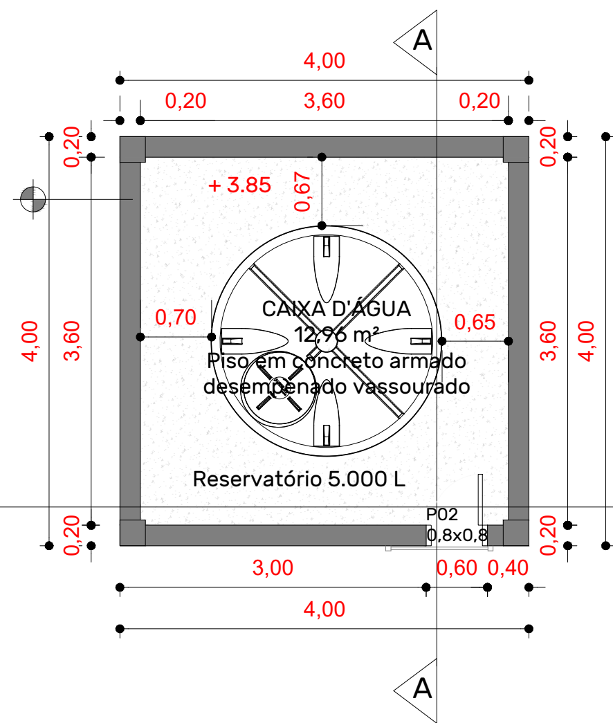
PLANTA - SUPERIOR (RESERVATÓRIO) ESC. 1:50
